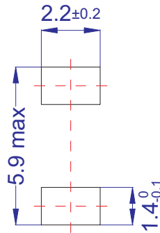
SMB DO-214 AA
