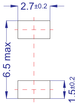
Melf DO-213 AB
