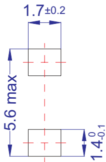
SMA DO-214 AC
