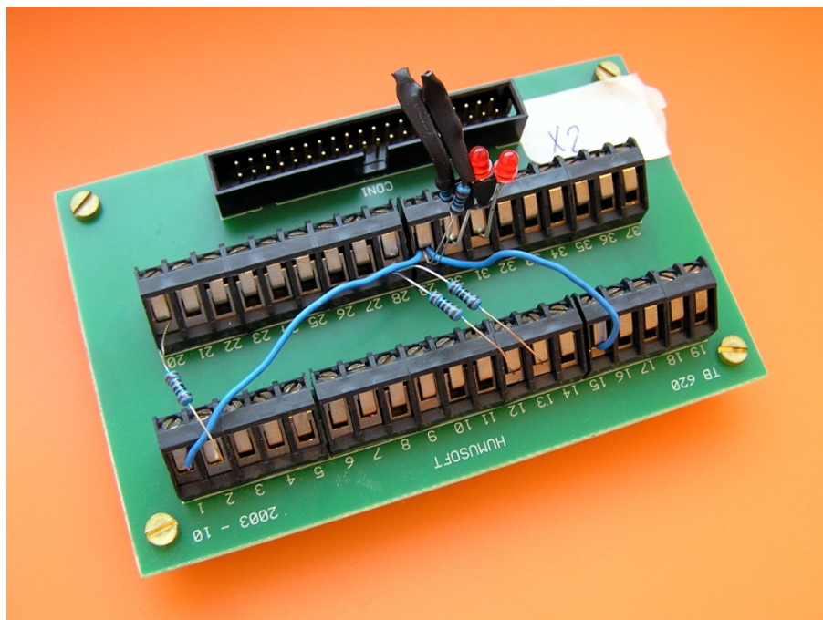
Obrázek 5.1: Svorkovnice TB620
